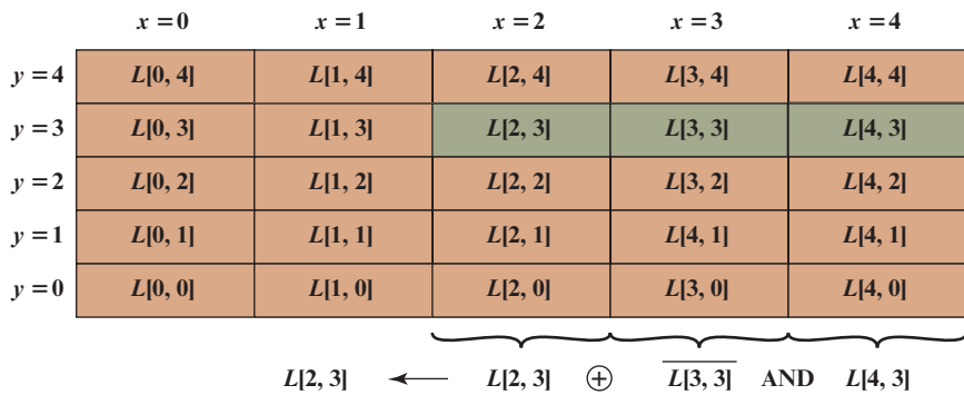
(b) \chi step function
